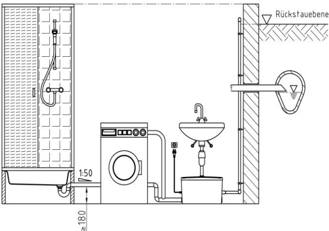
(Abb.2) Stecken Sie die Überwurfmutter (Pos. A), den Druckring (Pos. B) und den schwarzen Keil-Dichtring (Pos. C) wie abgebildet auf die DN 40-Abflussleitung und schieben Sie diese bis zum Anschlag in die Zulauföffnung des Behälters. Befestigen Sie die Abflussleitung, indem Sie die Überwurfmutter am Zulaufstutzen festdrehen, dabei muss der schwarze Keil-Dichtring zwischen Überwurfmutter und Zulaufstutzen liegen.
